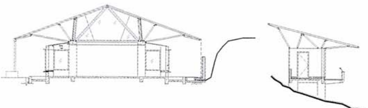
入口接待处剖面
